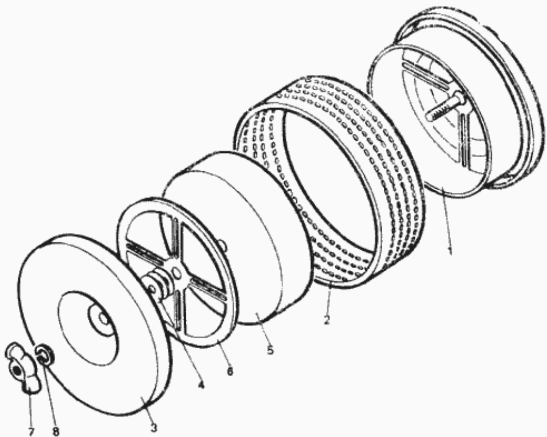
Рис. 59. Воздухоочиститель ПД8-1109012
